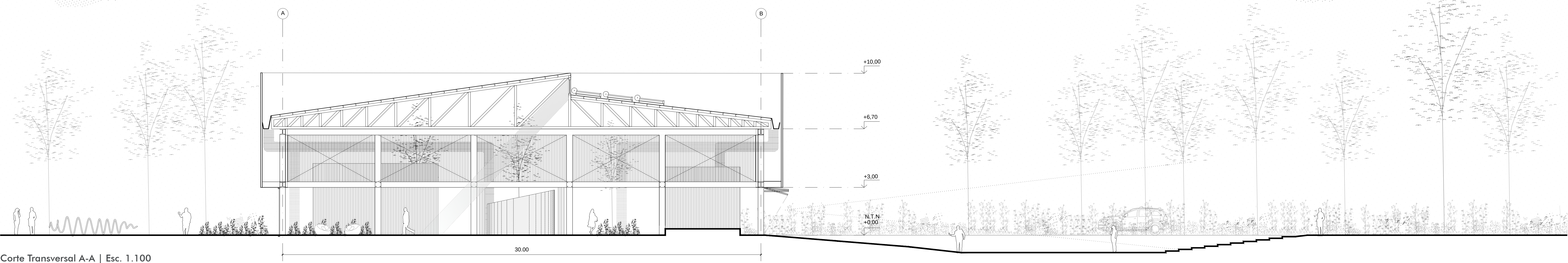
Corte Transversal A-A | Esc. 1.100
